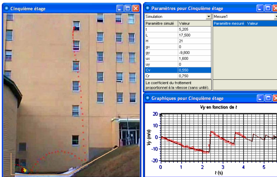
Figure 6. Comparaison du ballon réel et du ballon virtuel. Un ballon virtuel a été superposé à la séquence vidéo et les paramètres de simulation ont été ajustés afin de reproduire le mouvement filmé.
