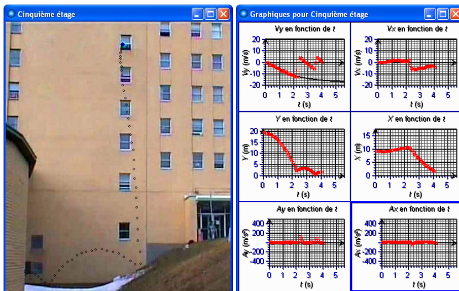
Figure 5. Mesures obtenues et graphiques produits pour la chute filmée d'un ballon. Les points sont mesurés en cliquant sur le ballon pour chacune des images de la séquence. Les graphiques sont générés automatiquement.
