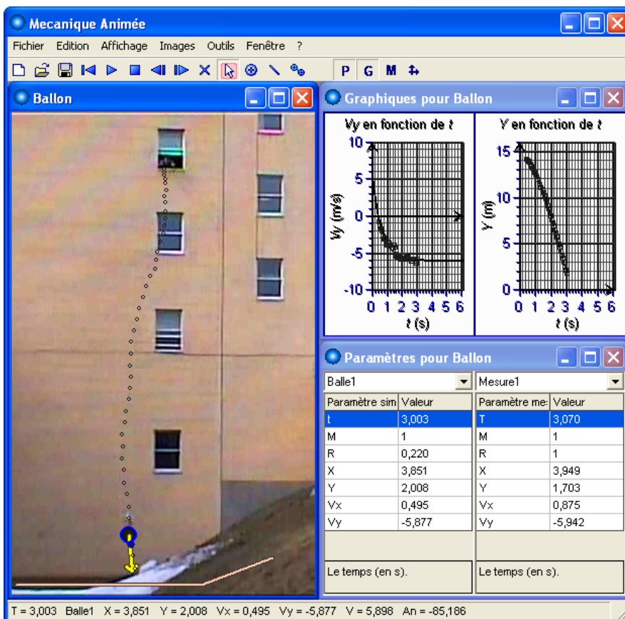
Figure 7. Copie d'écran typique obtenue lors des mises à l'essai systématiques. L'accélération du ballon n'est pas constante, une vitesse limite est obtenue à partir du graphique de V_y en fonction de t .
