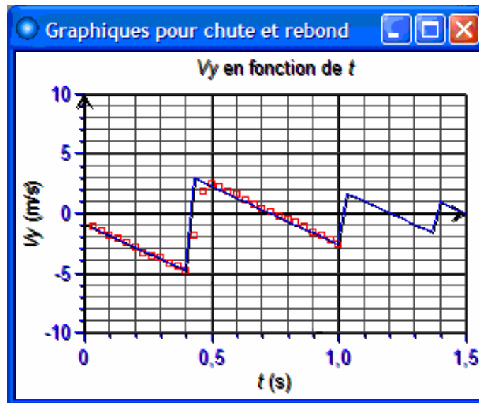
Figure 3. Exemple de fenêtre des graphiques illustrant la vitesse verticale d'une balle lors de sa chute et de ses rebonds : valeurs issues du film (petits carrés) et simulées (trait plein).
