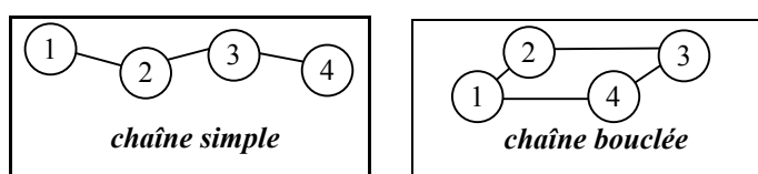
Figure 28. Chaînes de boules
