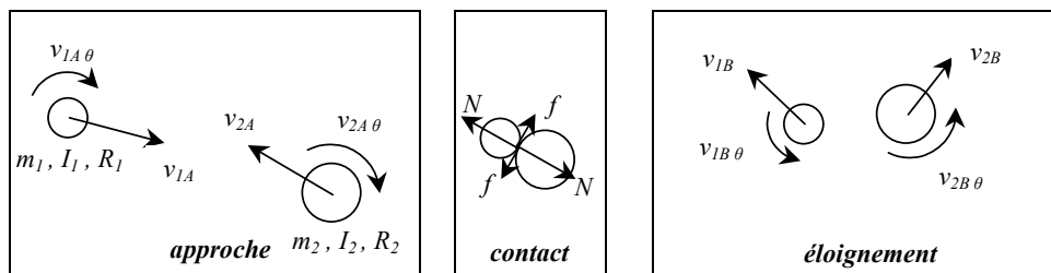
Figure 6. Collision entre deux boules
