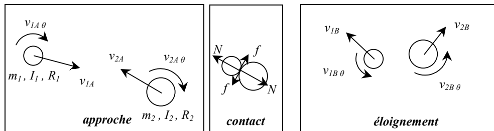
Figure 27. Collision entre deux boules
